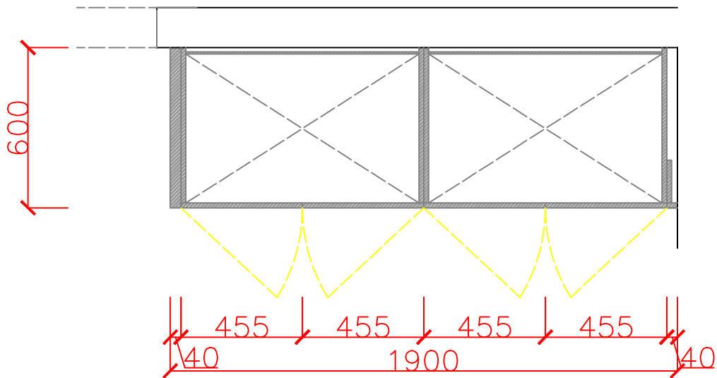
Grondplan
