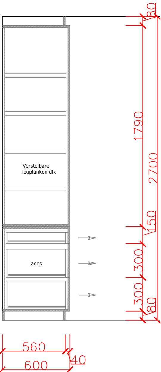
Doorsnede
