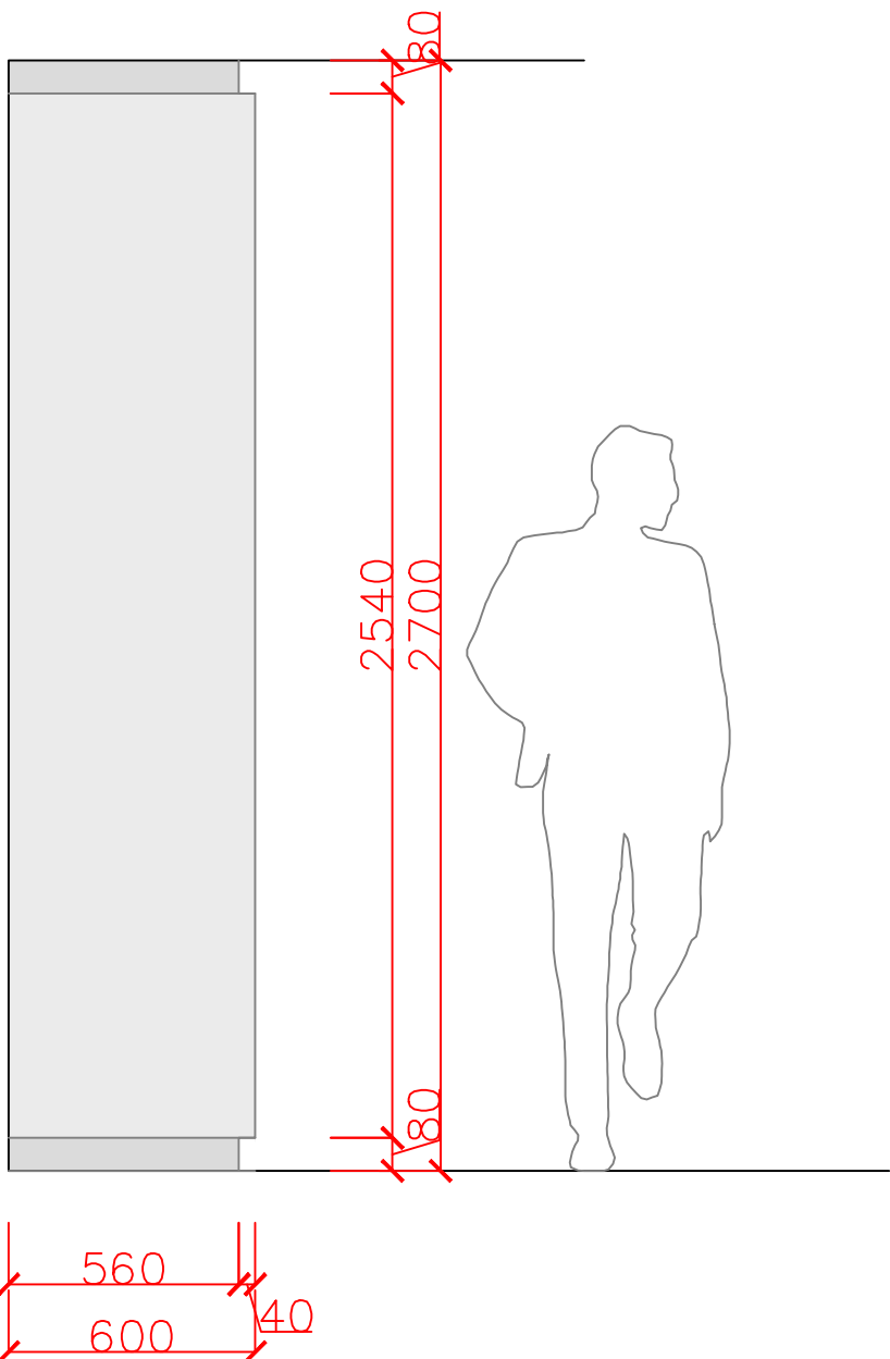
Zijaanzicht
