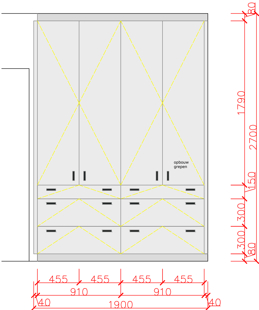
Kastindeling
