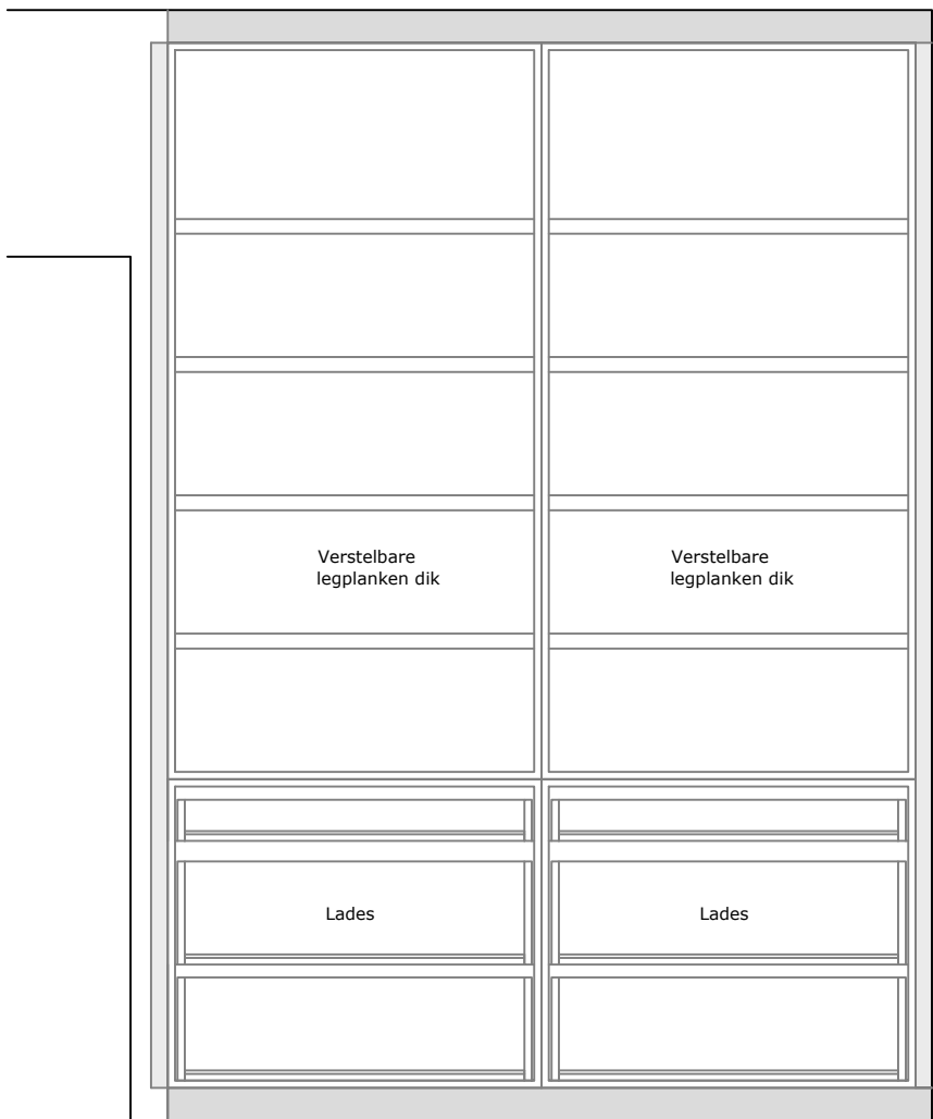
Kastindeling
