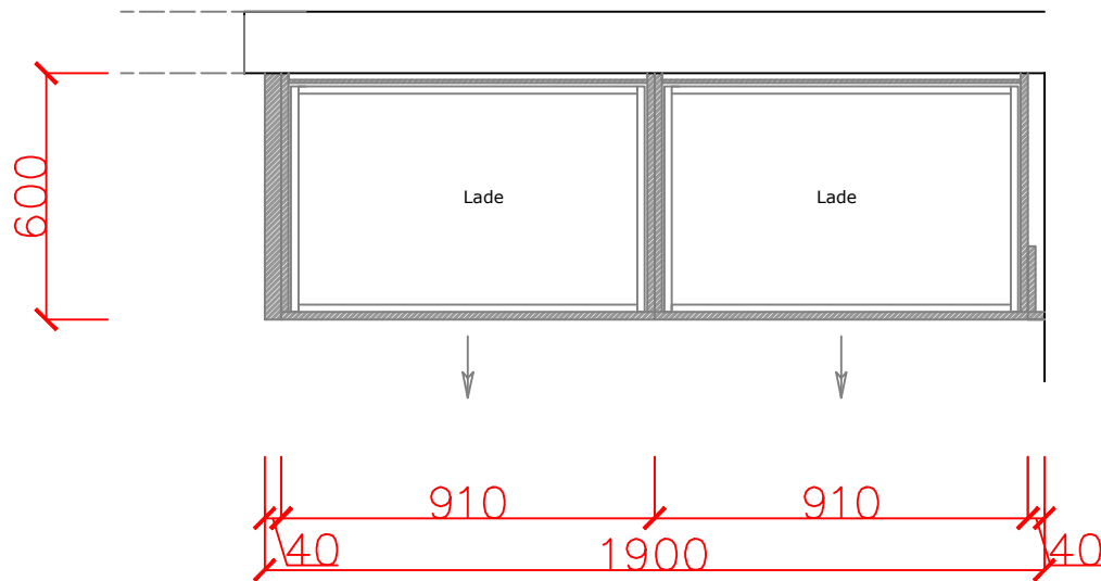
Grondplan onderkasten
